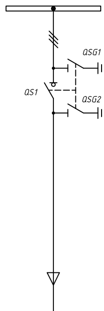
Схема 4 – Ячейка с выключателем нагрузки и двумя заземляющими ножами
