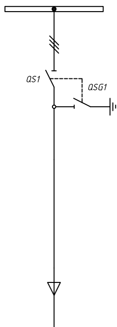
Схема 1 – Ячейка с разъединителем и заземляющим ножом
