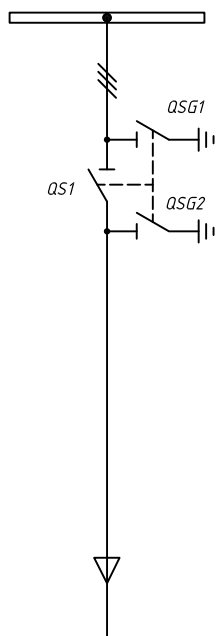
Схема 3 – Ячейка с разъединителем и двумя заземляющими ножами
