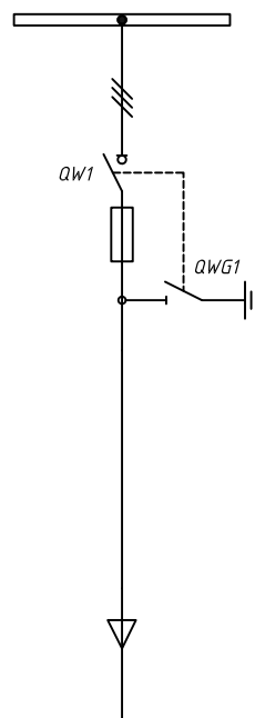
Схема 2 – Ячейка с выключателем нагрузки, плавким предохранителем и заземляющим ножом
